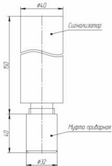
Рисунок 37 - Пневматический звуковой сигнализатор
