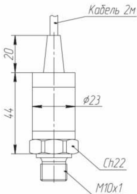
Рисунок 4 - Преобразователь (датчик) давления
