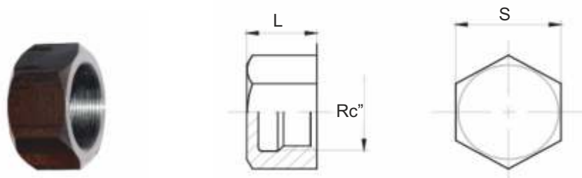
Рисунок 40 - Заглушка для установки на выпускном трубопроводе на ниппели
