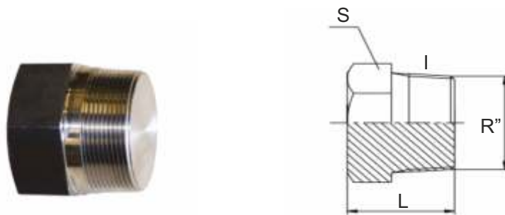
Рисунок 41 - Заглушка для установки на выпускном трубопроводе вместо РВД
