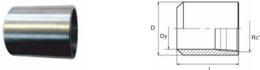
Рисунок 11 - Муфта переходная
